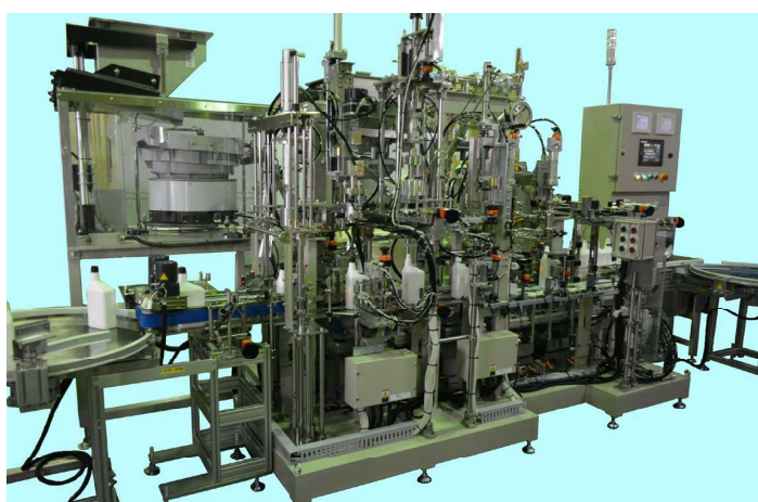
■ 多種容器兼用自動充填・蓋締機 (1L～5L/丸缶・角缶/打栓・スクリュー栓)
