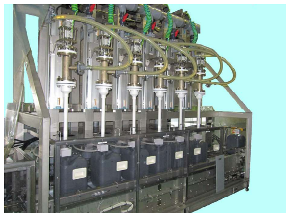
■ 6連自動充填機 (液面追従式) (テフロンバルブ)
